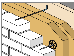
Монтаж базальтопластиковых связей Terlo-L-Tie
