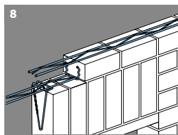
8 Арматура Murfor RND/Z-50 во втором ряду кладки. Далее по высоте 1 арматура каждые 300...500 мм
